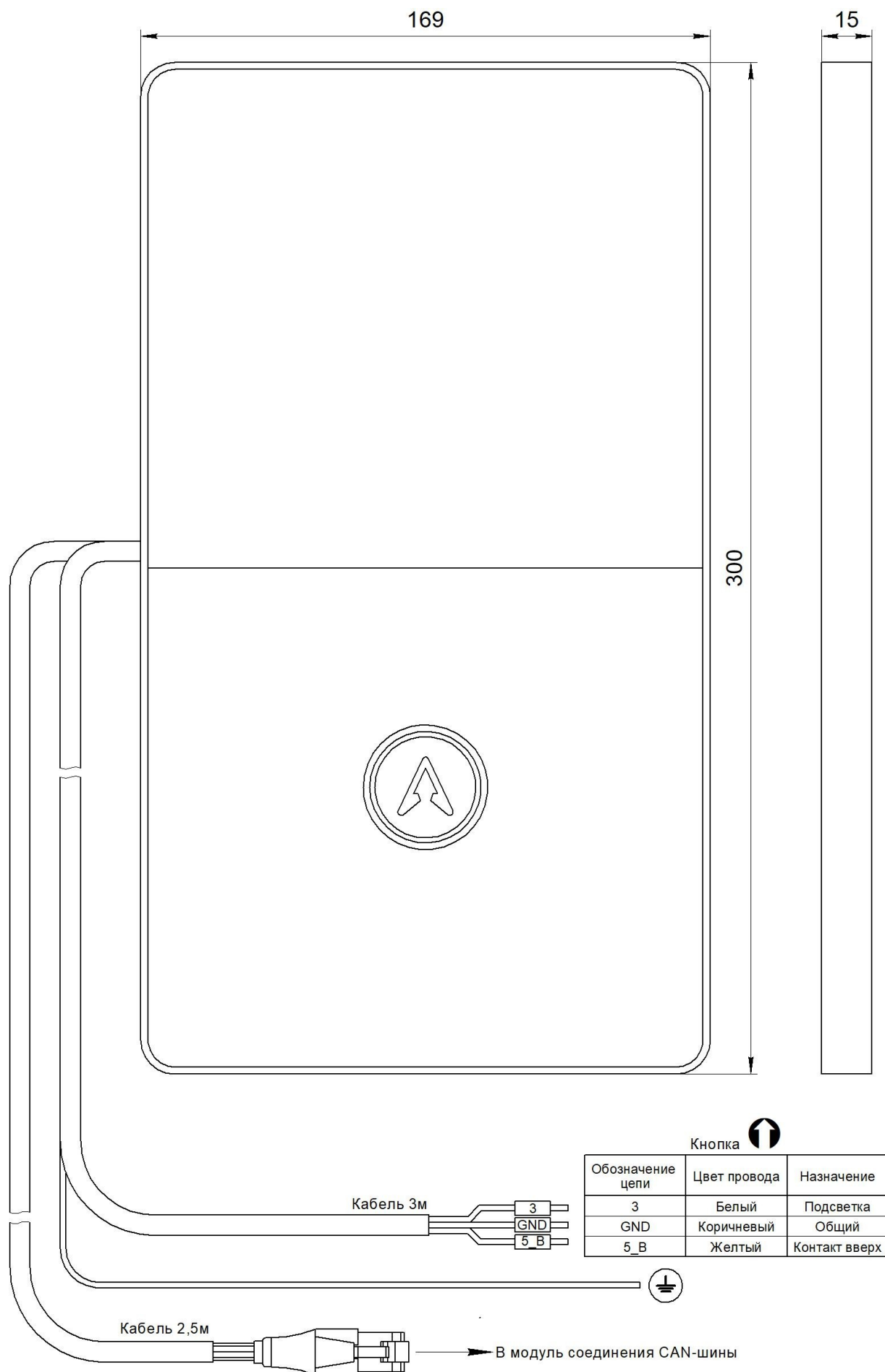
Рис.1 Внешний вид Вызывной пост ОНИКС (жгут RJ45) НШЕК.468381.023
